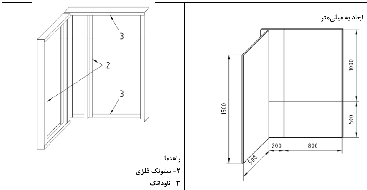
شکل ب-۱-ب زیرسازه
