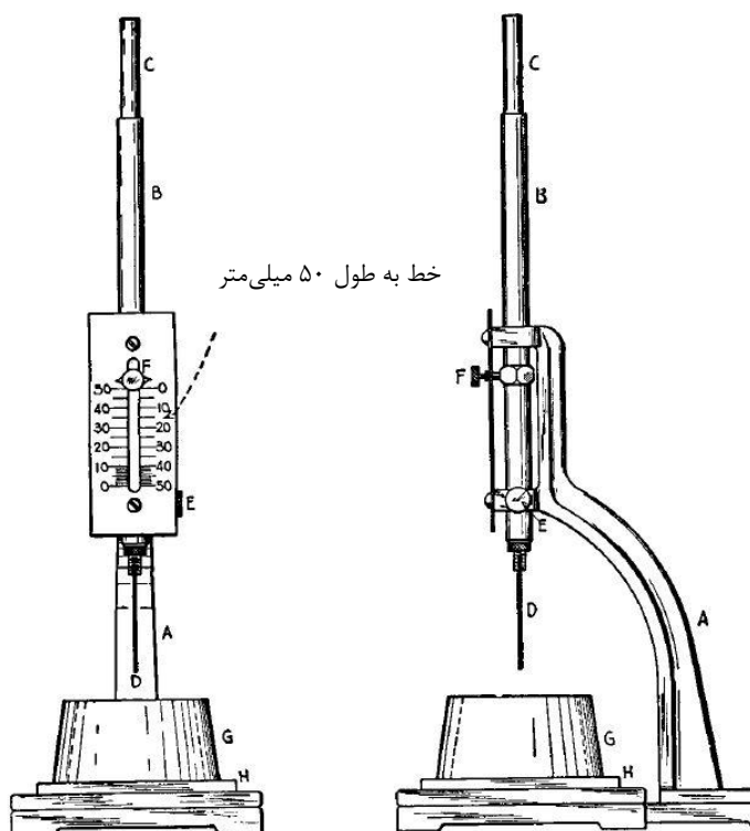
شکل ۳- دستگاه ویکات
